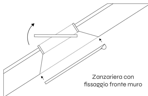
FIGURA 2 SEZIONE LATERALE
