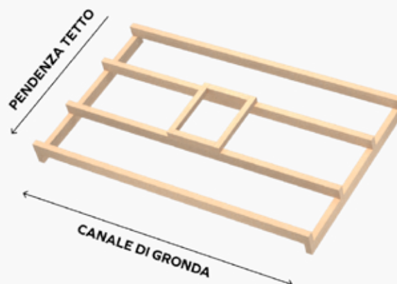
FIGURA 2 - Travi con orditura orizzontale
