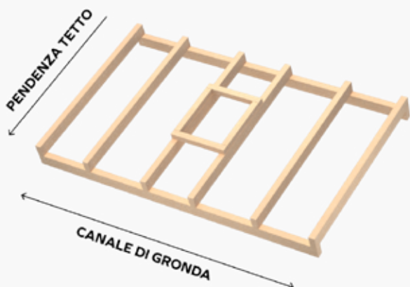
FIGURA 1 - Travi con orditura verticale
